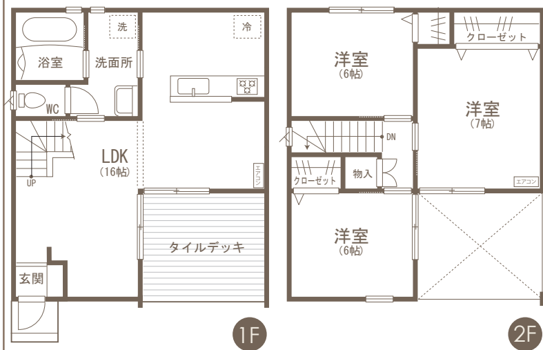
間取図 (C・D棟共通)
